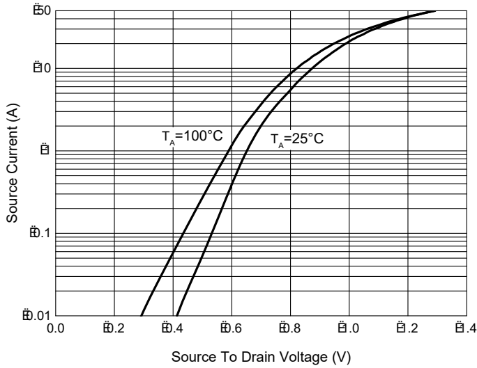
Fig. 7 - I_S - V_{SD}
