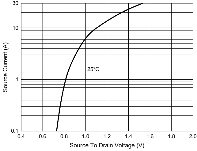
Fig. 7 - I_S - V_{SD}
