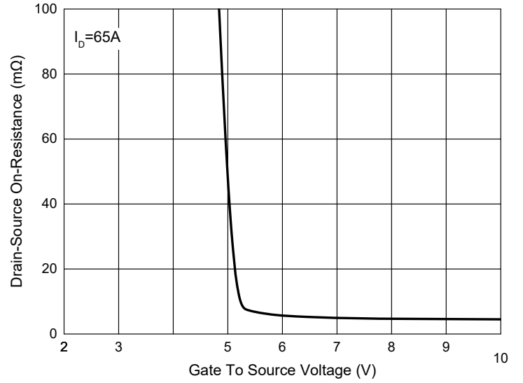
Fig. 8 - R_{DS(ON)} - V_{GS}
