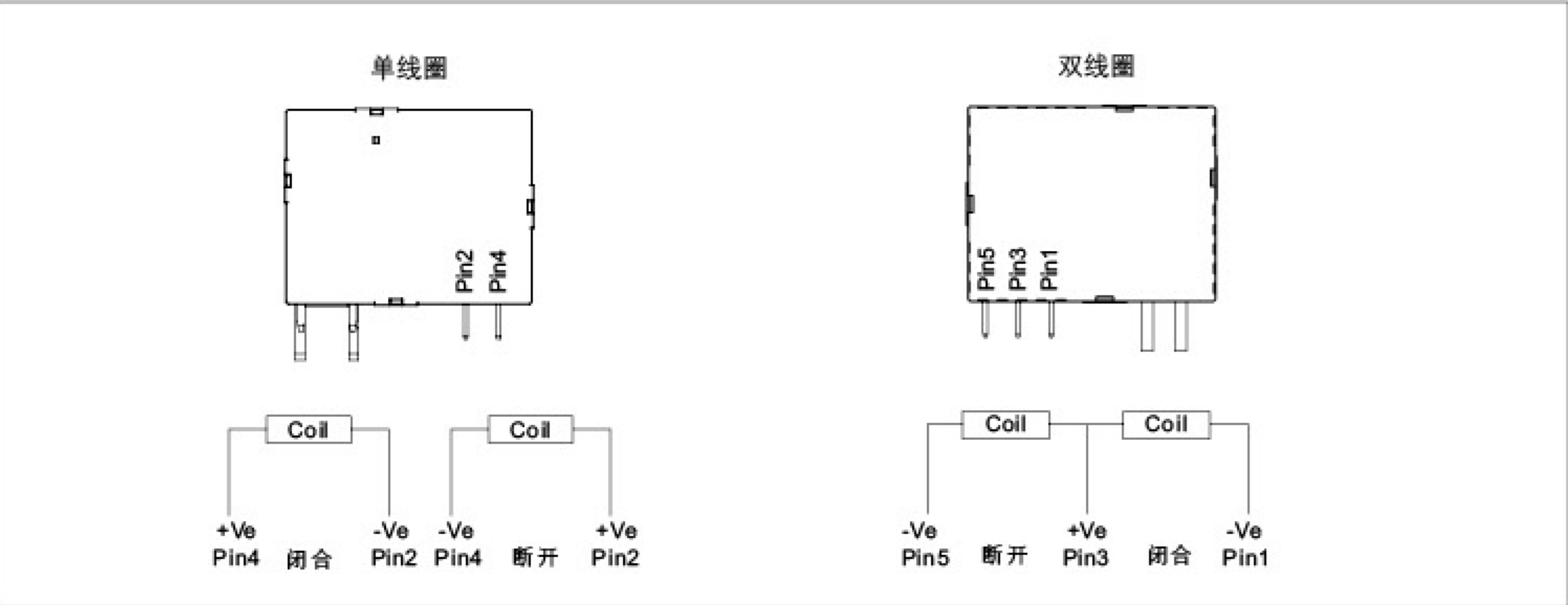
接线图
