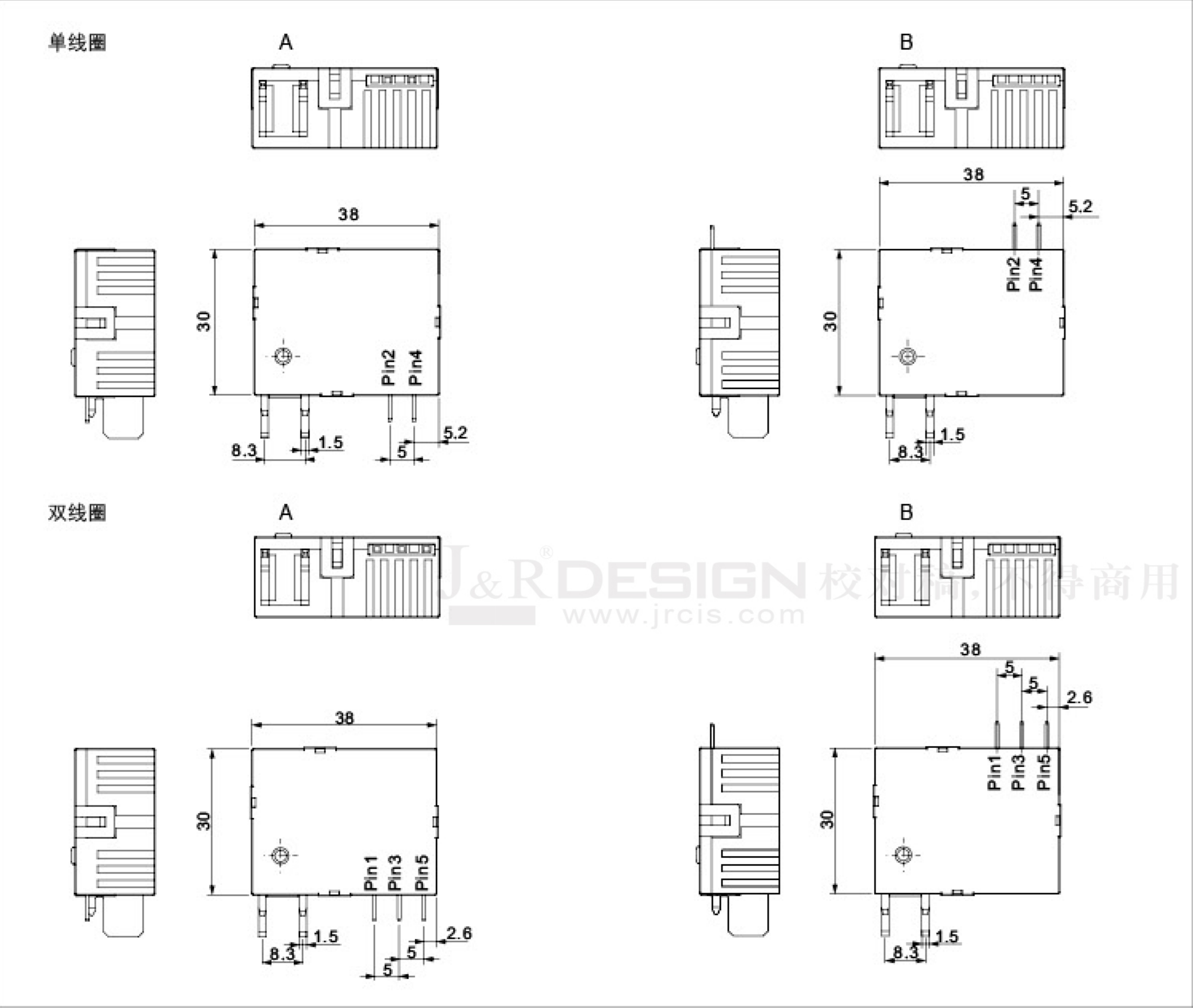
外形尺寸图
