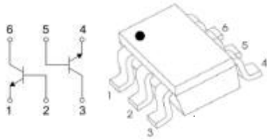
SOT-363
