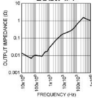
输出阻抗-频率
