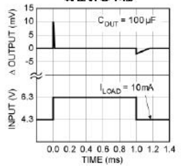
线性瞬态响应
