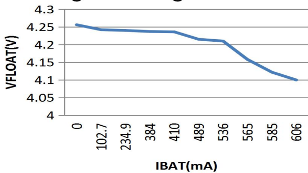
浮充电压与充电电流关系
