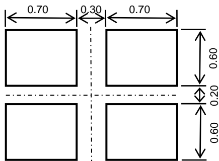
第1図 外形寸法図
