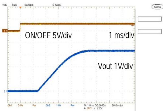
On/Off Enable Delay (Vin=12V, Vout=3.3V, Iout=4A, Cload=400uF)
