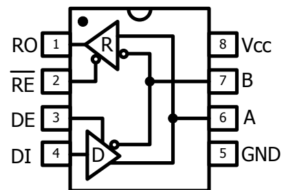
MX485E
