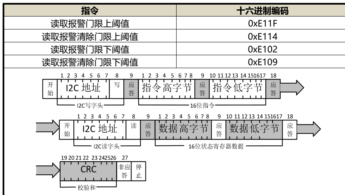
图 12.13-1 读取警报门限指令 (白色块由微控制器控制, 传感器响应为灰色块)
