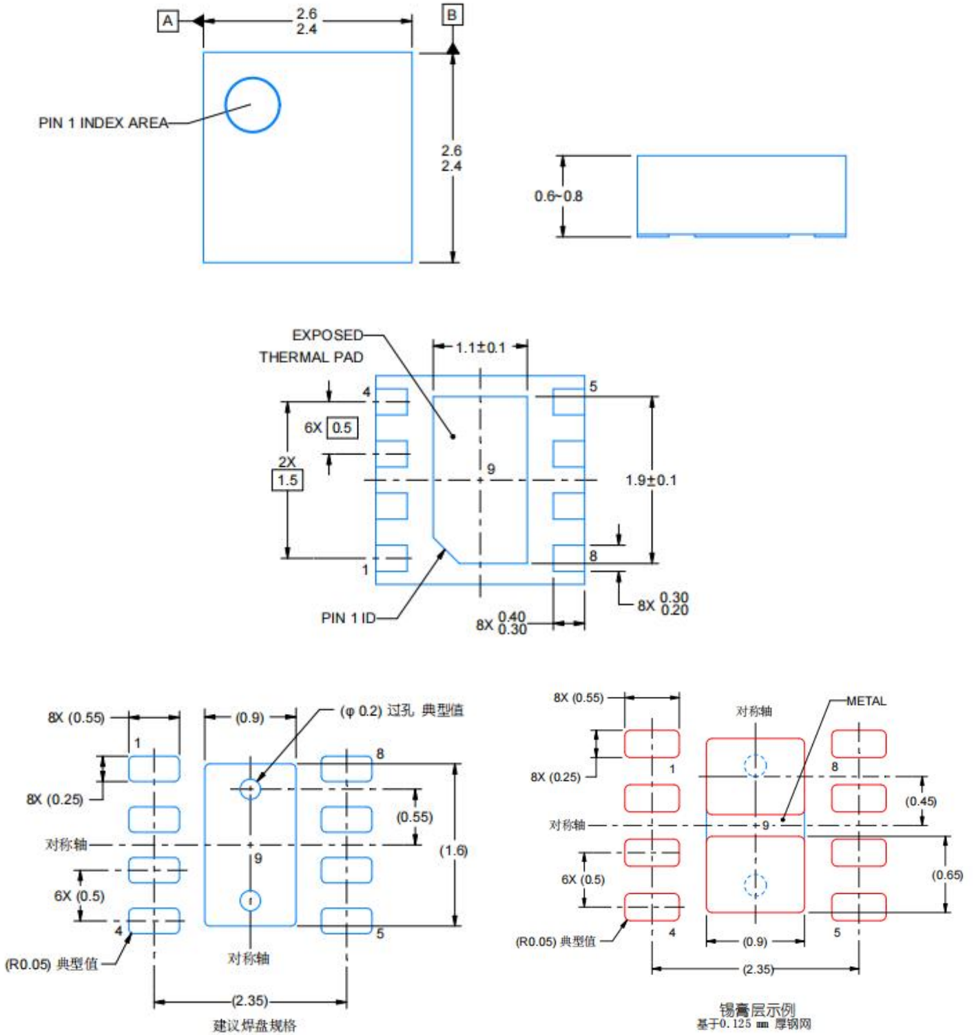
图 13.2 PCB 焊盘引脚尺寸图
