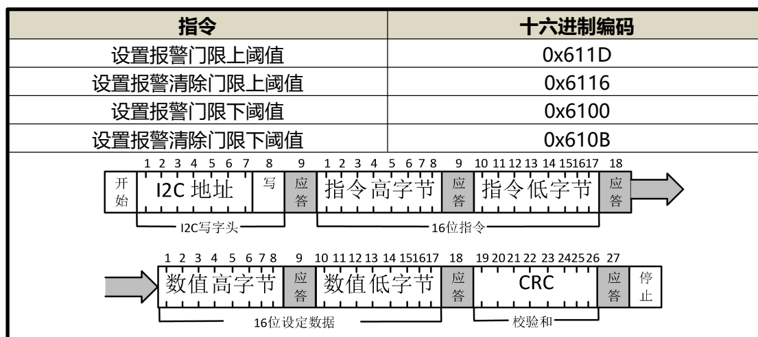
图 12.13-2 写入警报门限指令 (白色块由微控制器控制, 传感器响应为灰色块)
