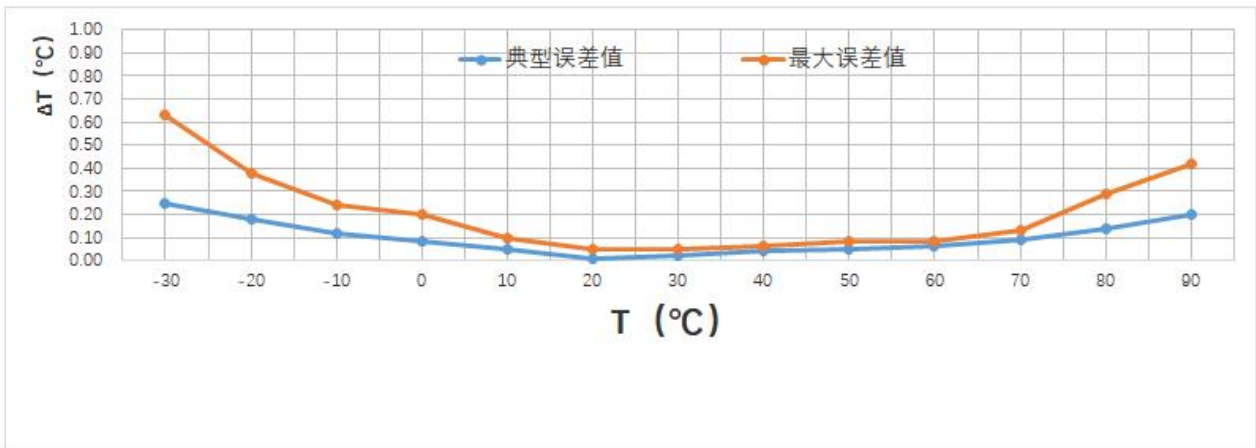
图 7- 3 MTS01W 精度误差曲线
