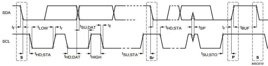
图 12.15 I 2 C 时序参数
