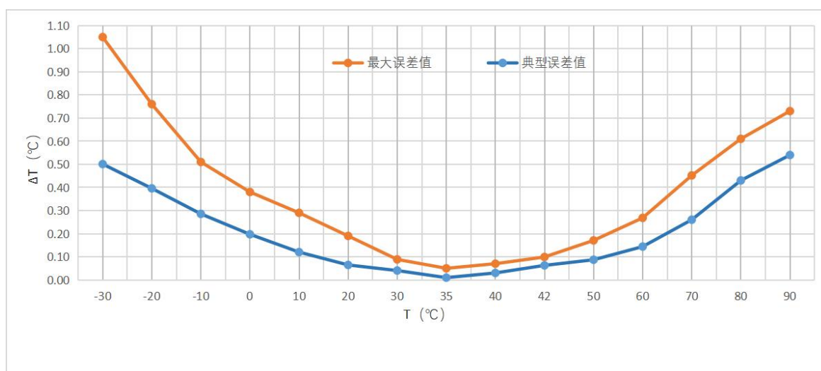
图 7- 1 MTS01 精度误差曲线
