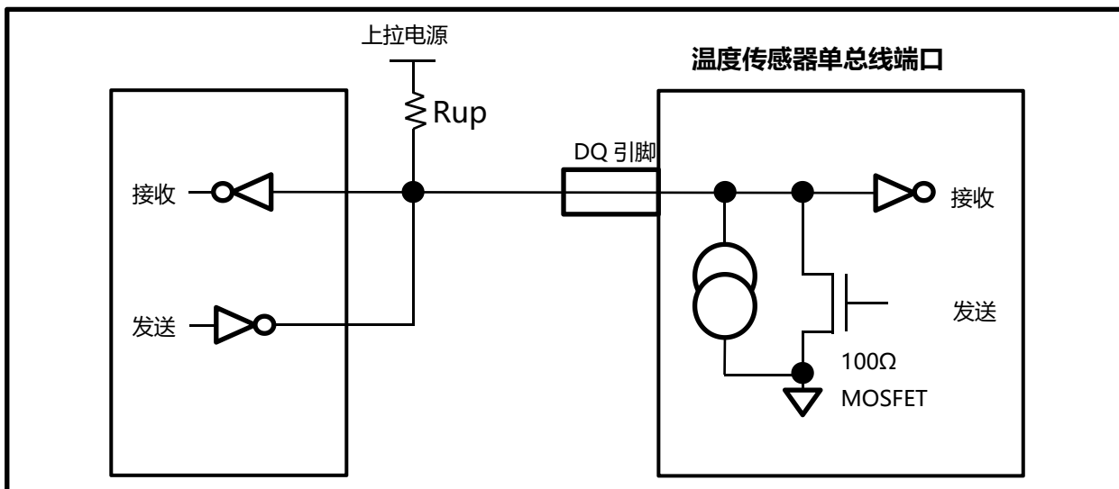
图 11.1 单总线硬件配置
