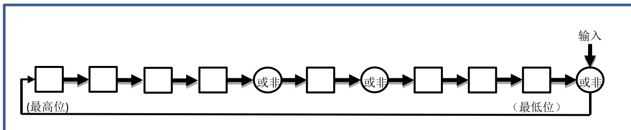
图 11.2 循环冗余校验生成器
