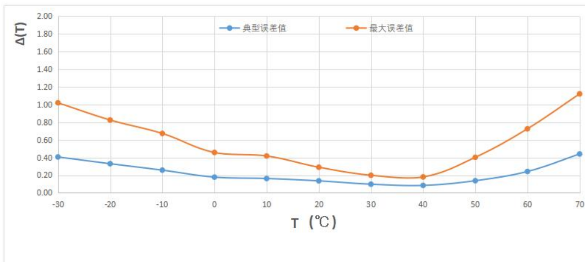
图 7- 5 MTS01B 精度误差曲线
