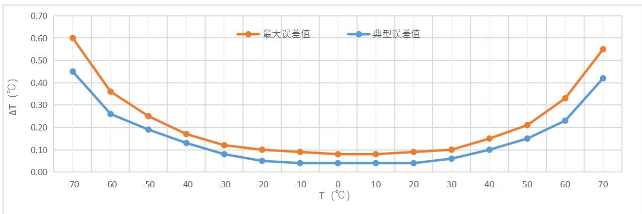
图 7- 4 MTS01P 精度误差曲线
