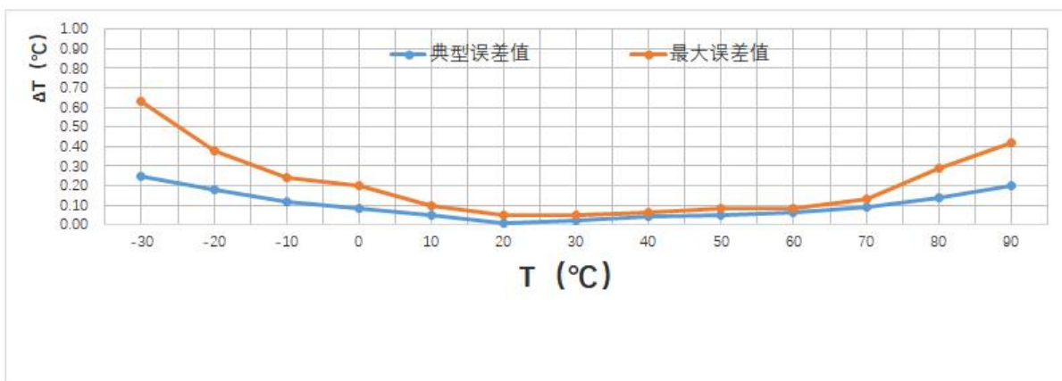
图 7-2 M117Z 精度误差曲线
