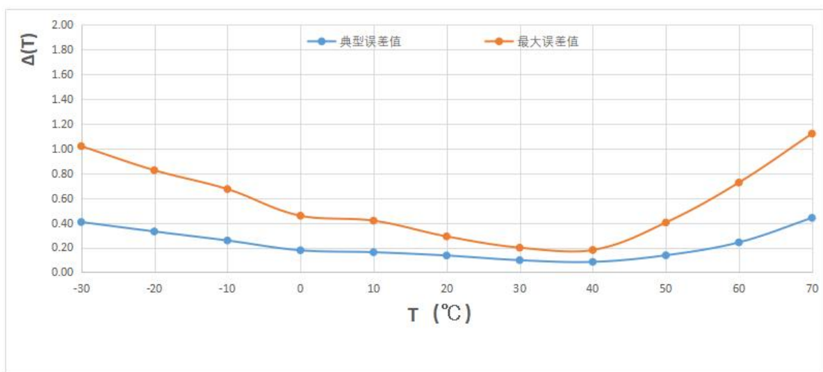
图 7-5 M117B 精度误差曲线
