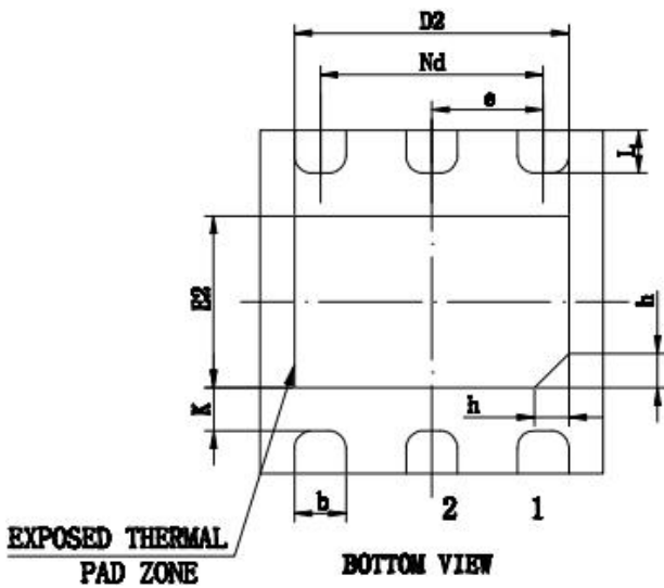
封装尺寸图 DFN6L(2X2X0.75mm)
