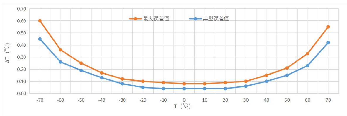
图 7-4 M117P 精度误差曲线
