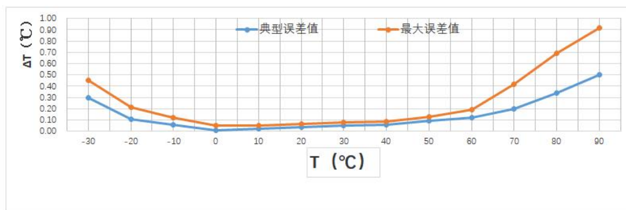
图 7-2 M117Z 精度误差曲线
