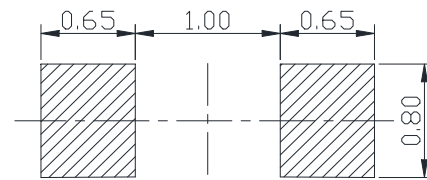
推荐焊盘尺寸
