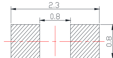
推荐焊盘尺寸
