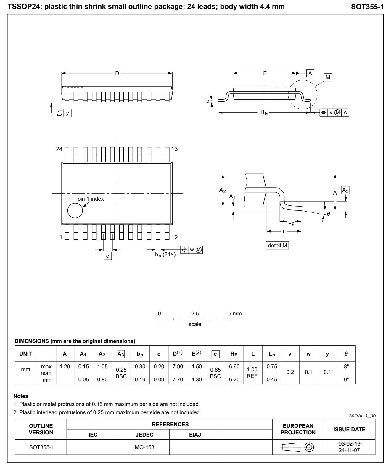
Fig. 14. Package outline SOT355-1 (TSSOP24)
