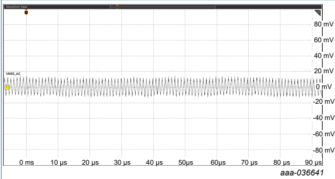
Fig. 23. V_{NEG} output ripple ( I_{NEG} = 80 mA)
