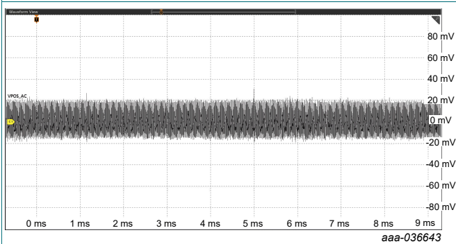
Fig. 25. V_{POS} output ripple ( I_{POS} = 40 mA)
