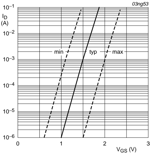
T_j = 25^\circ\text{C}; V_{DS} = V_{GS}
