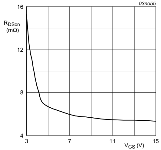
T_j = 25^\circ\text{C}; I_D = 25\text{A}
