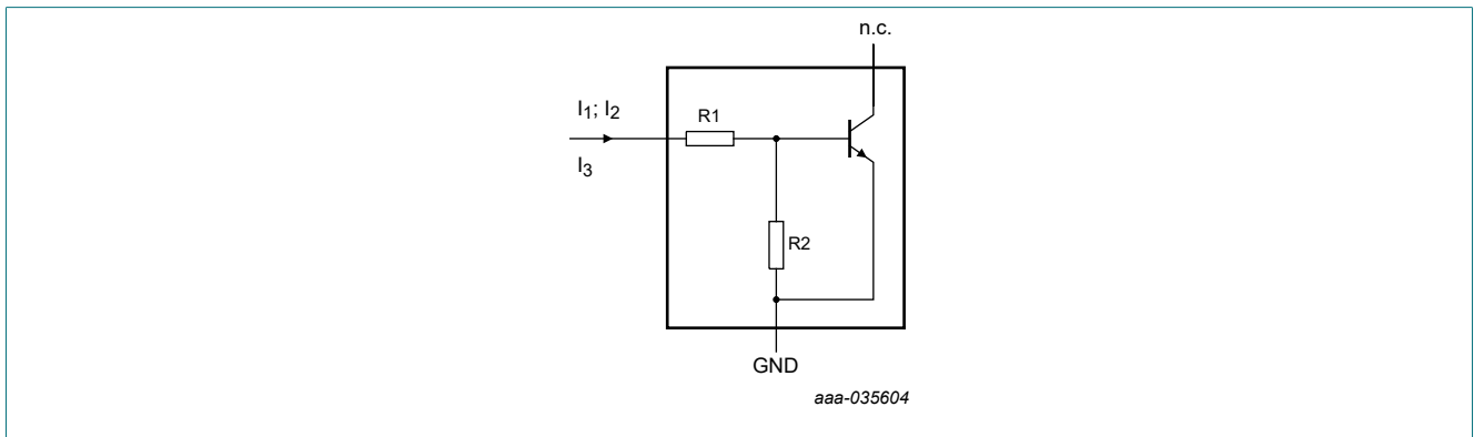
Fig. 15. TR1 (NPN): Resistor test circuit
