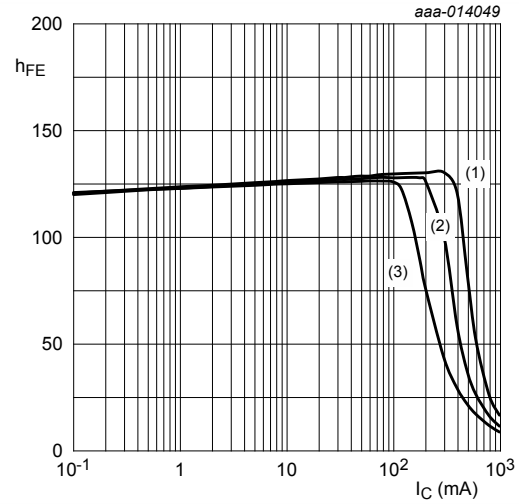
T_{amb} = 25\text{ }^\circ\text{C} (1) V_{CE} = 10\text{ V} (2) V_{CE} = 25\text{ V} (3) V_{CE} = 50\text{ V}
