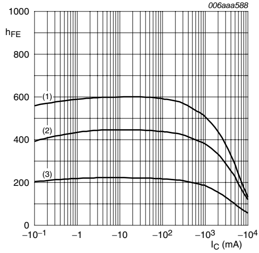
V_{CE} = -2 V (1) T_{amb} = 100^\circ C (2) T_{amb} = 25^\circ C (3) T_{amb} = -55^\circ C
