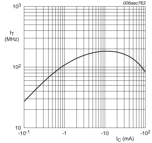
V_{CE} = -5\text{ V}; T_{amb} = 25\text{ }^{\circ}\text{C}
