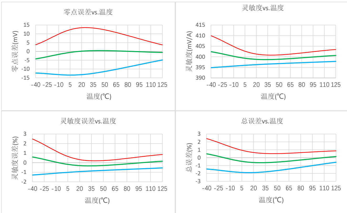
[1] 绿色代表平均值，红色线代表平均值+3Sigma，蓝色线代表平均值-3Sigma，在-40°C，25°C，125°C下测量拟合得出。
