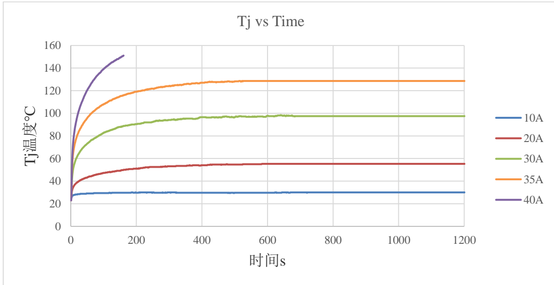
Figure 6.4 NSM2012 在不同电流下结温曲线
