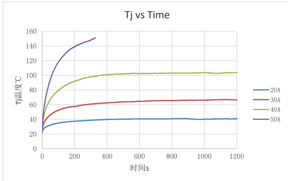
Figure 6.3 NSM2015 在不同电流下结温曲线
