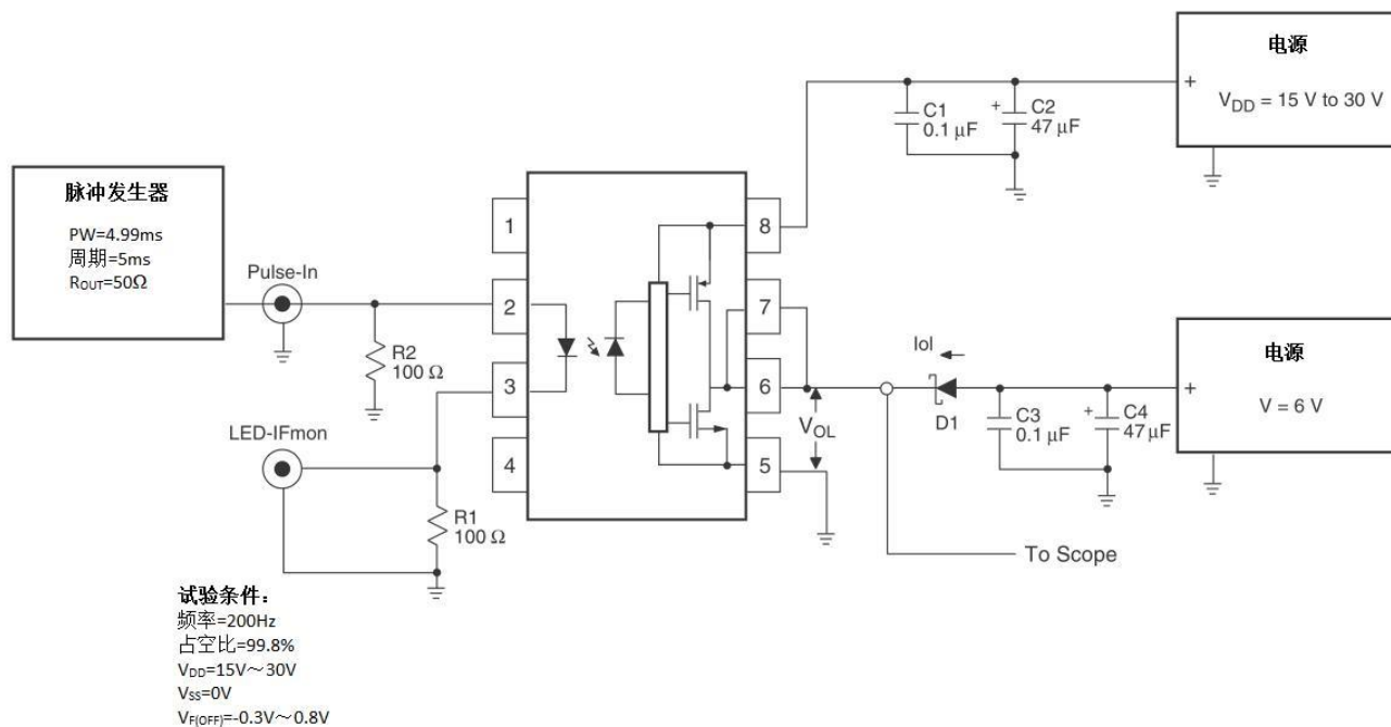
I_{OL} 测试电路
