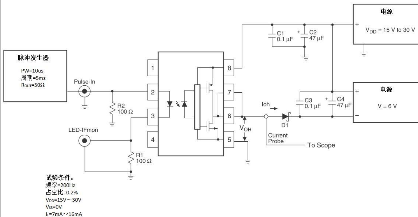
I_{OH} 测试电路
