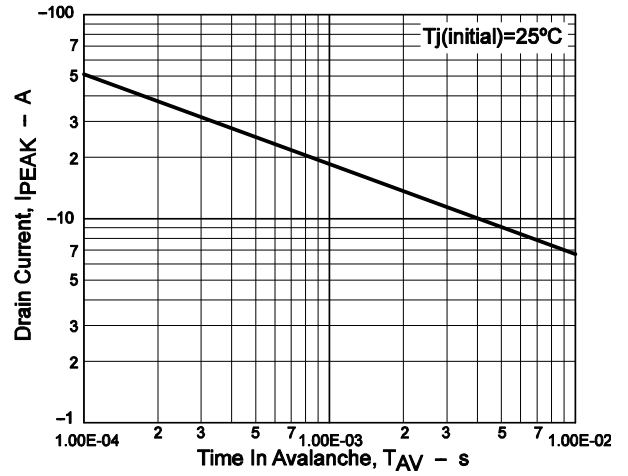
Figure 10. I PEAK - T AV
