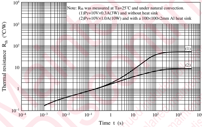
R_{th} - t
