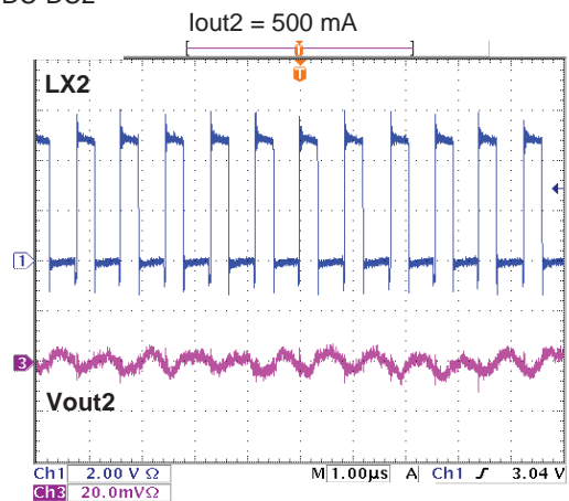
DC-DC2
