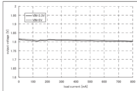
DC-DC2
