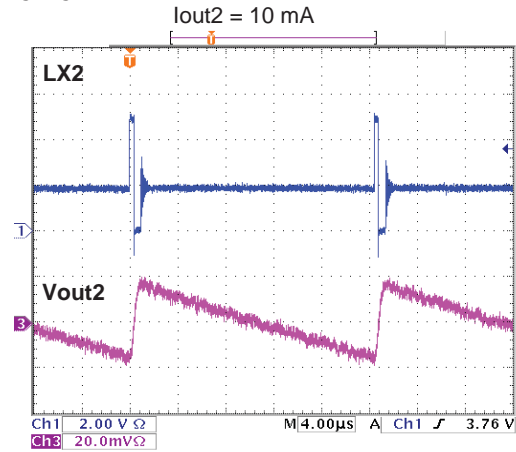
DC-DC2
