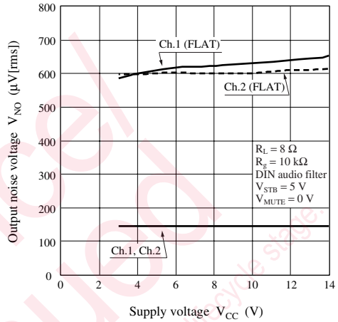
V_{NO} — V_{CC}
