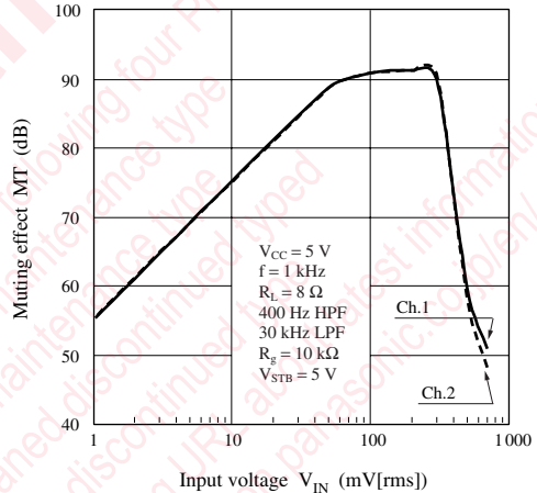
MT — V_{IN}
