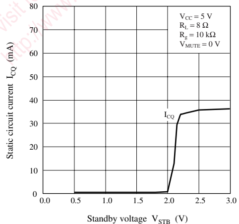
I_{CQ} — V_{STB}
