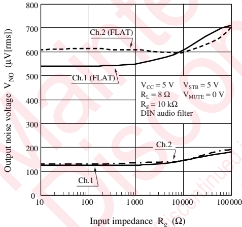
V_{NO} — R_g
