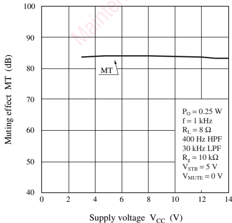
MT — V_{\text{CC}}
