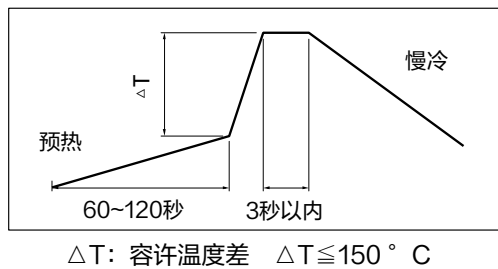
烙铁焊接标准模式 (例)
