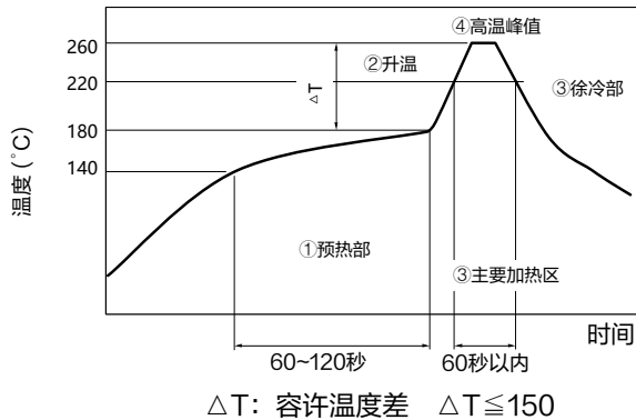
回流焊推荐模式 (例)
