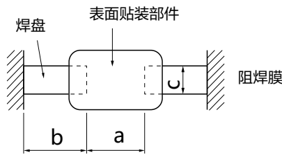
推荐焊盘尺寸 (例)
