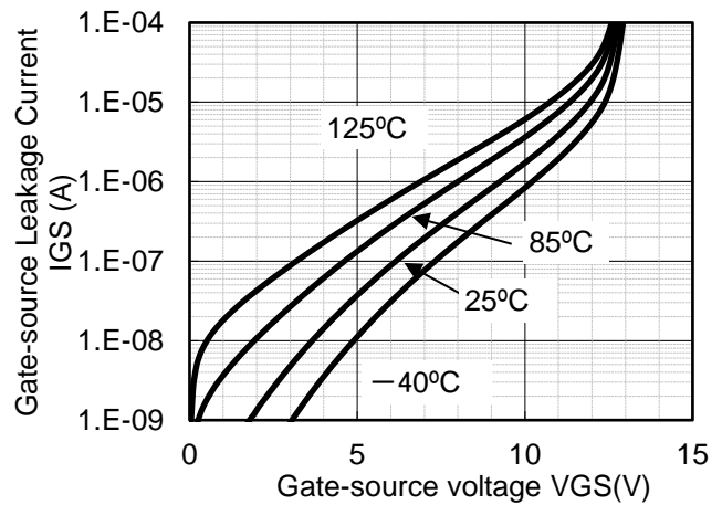
IGS - VGS
