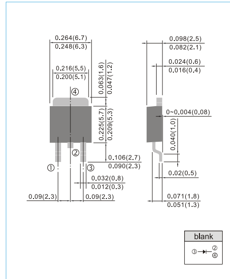
TO-252 Unit : inch(mm)
