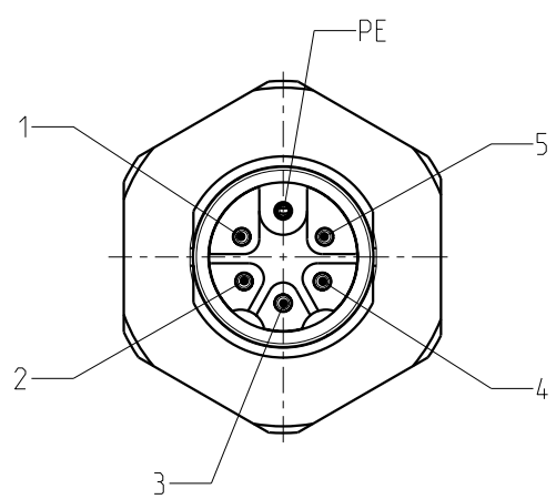
6pol M-Codierung (Steckseite) / 6pole M-coding (plug-in side)
