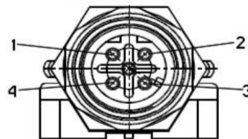
Ansicht X
