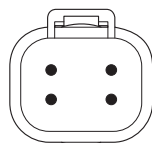
DEUTSCH DT04-4P pin assignment
