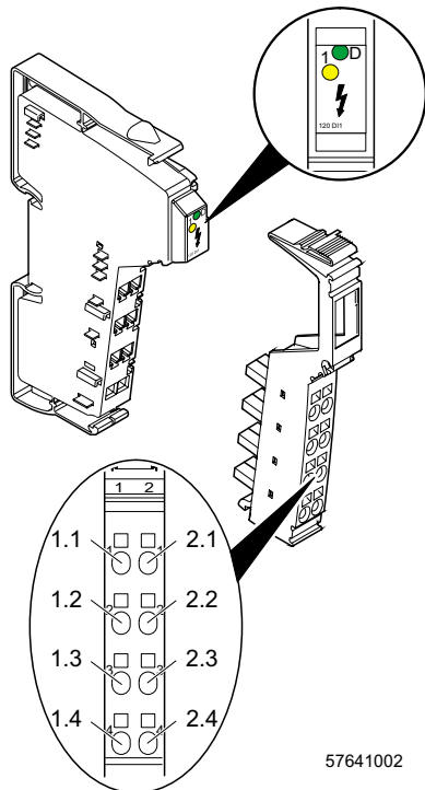
Figure 2 IB IL 120 DI 1 with the appropriate connector
