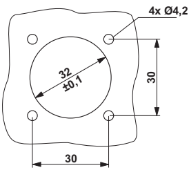
Installation dimensions SM-...PWN8AWA00
