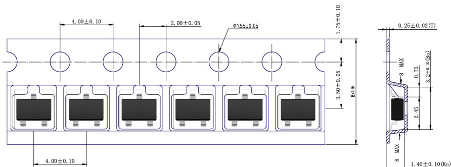
SOT-23-3
