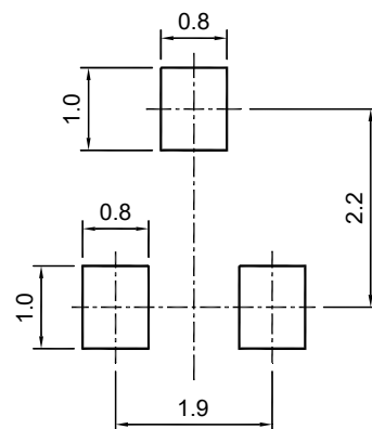
SOT-23
