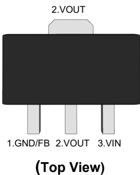
SOT-89
