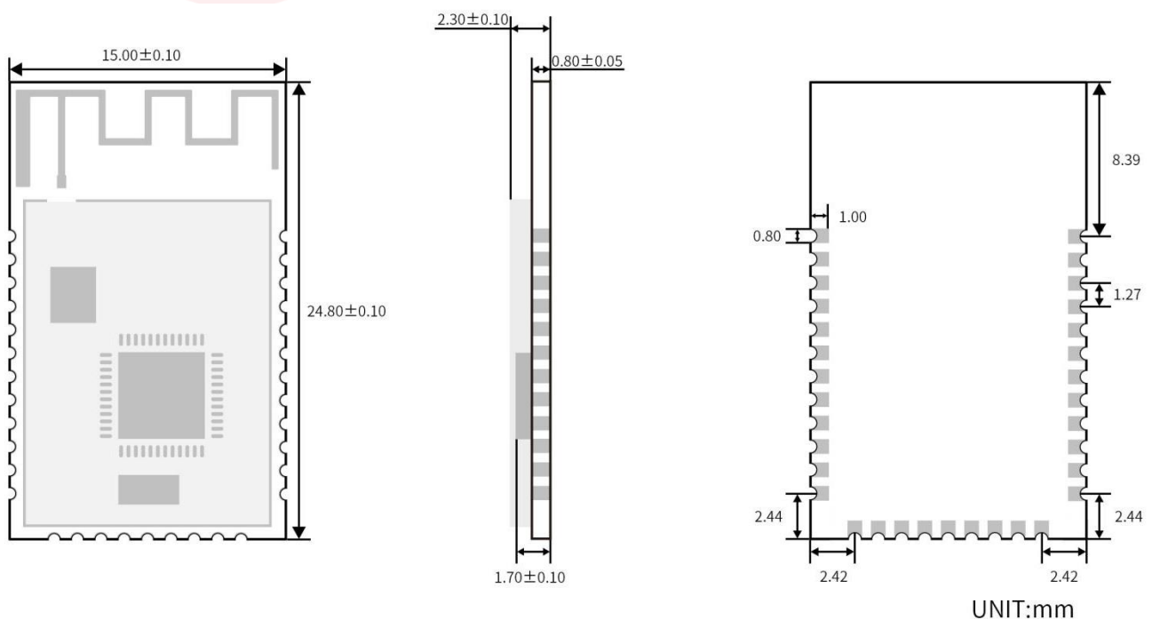
图 2. RF-BM-ND04尺寸图
