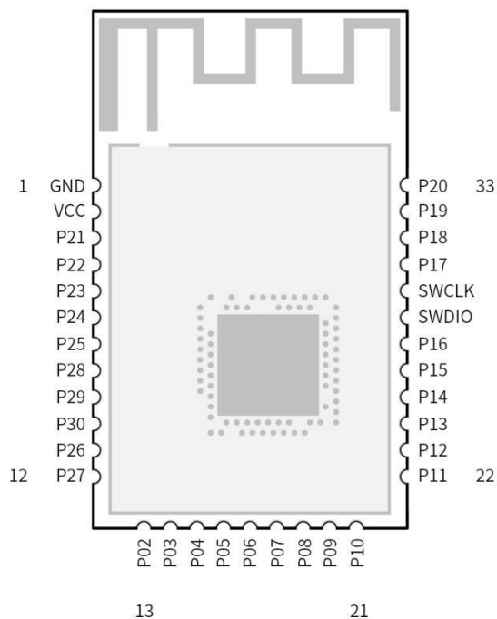
图 3. RF-BM-ND05引脚图
