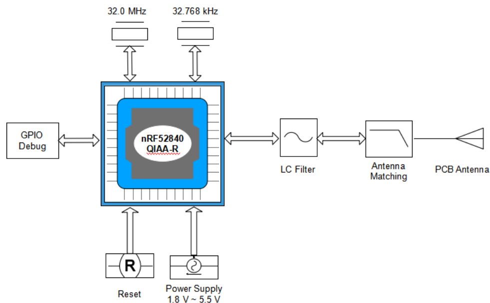
图 1. RF-BM-ND05 原理框图
