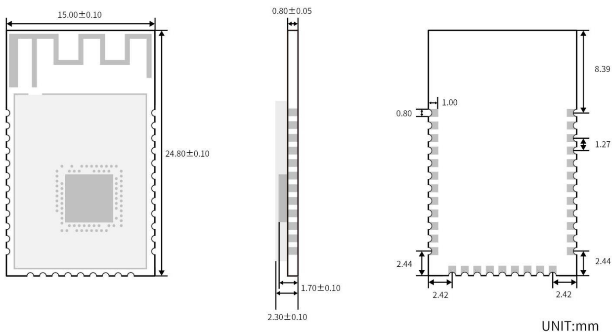
图 2. RF-BM-ND05尺寸图
