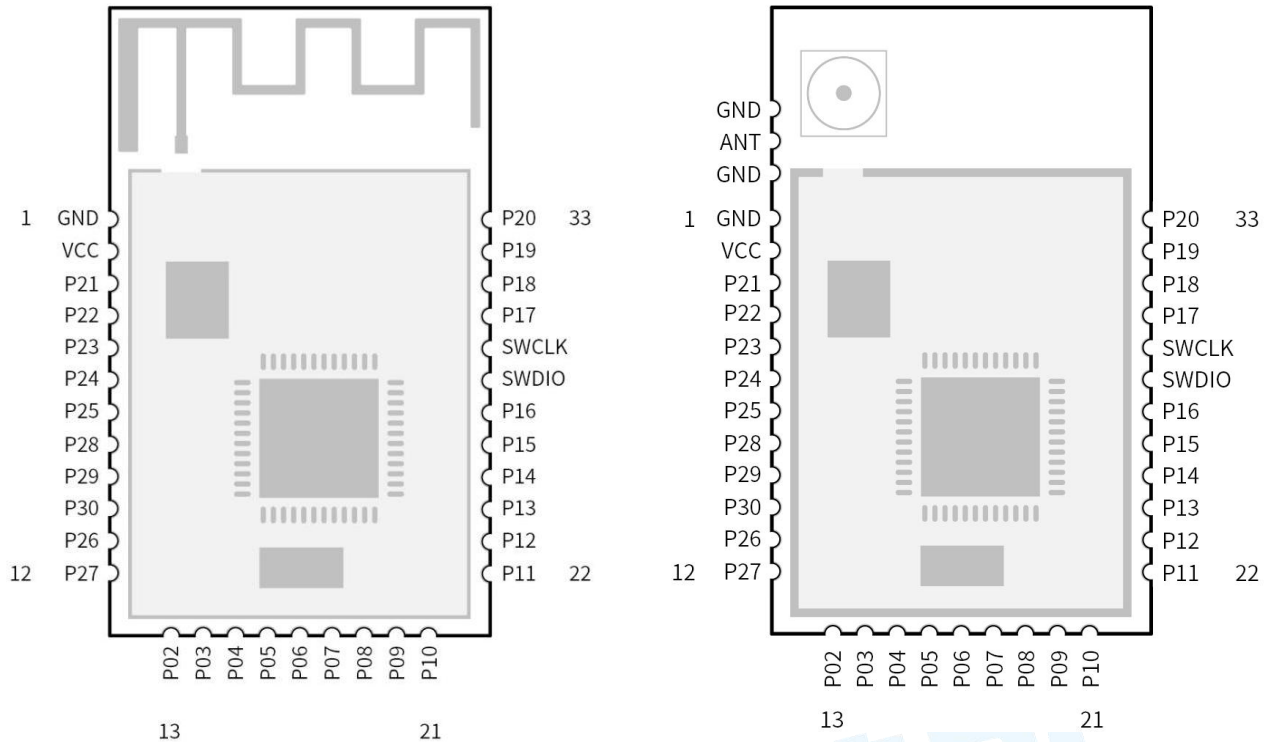
模块引脚图
