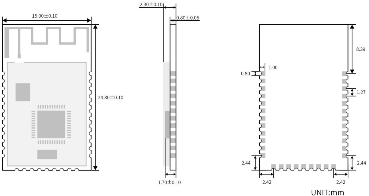
图 2. RF-BM-ND04C 尺寸图
