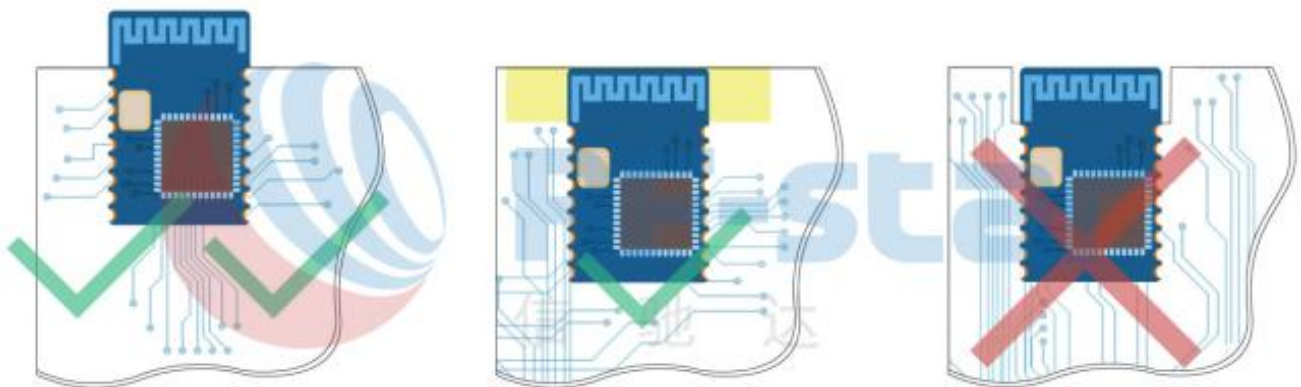
图 5. 布局建议
