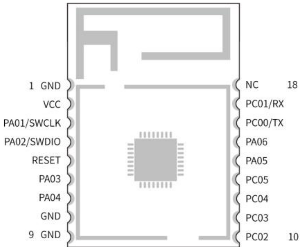
引脚定义图
