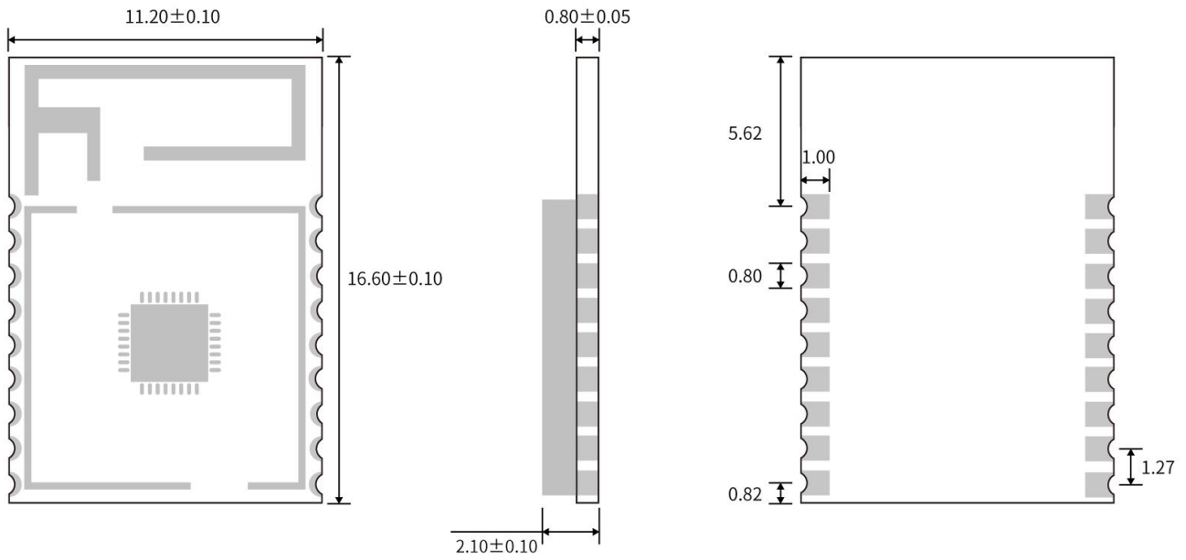
RF-BM-BG22B1\B2\B3 尺寸图
