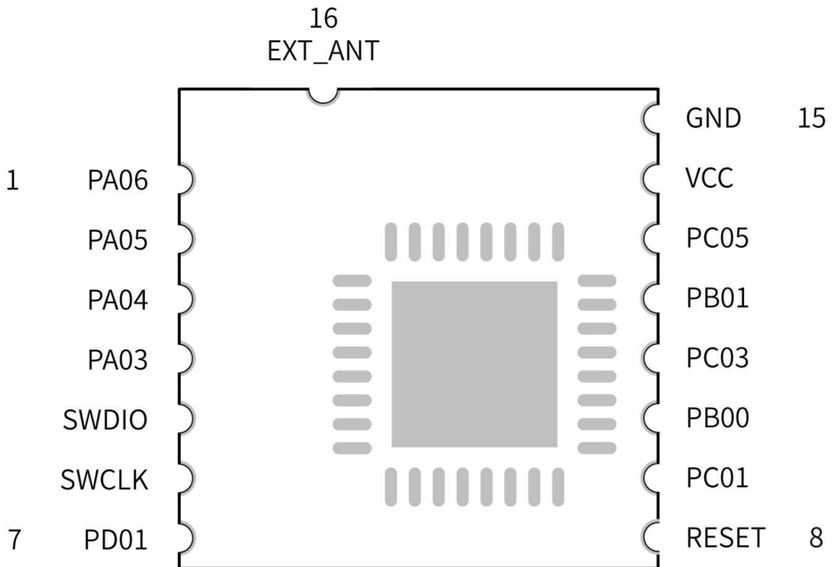
图 3. 引脚图
