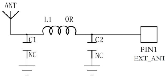
图 6. 外置天线设计原理图
