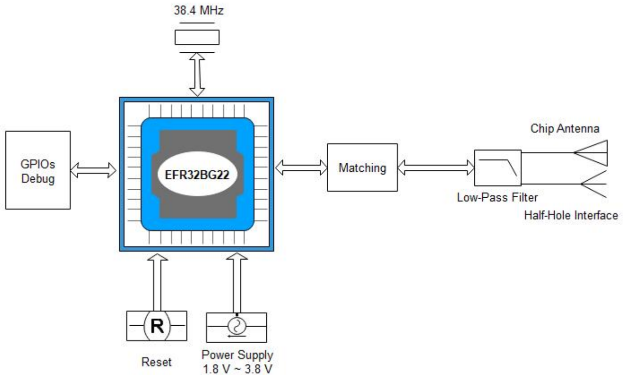
图 1. 原理框图
