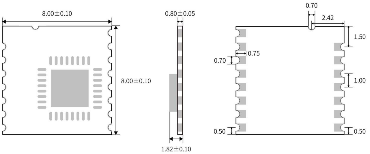
图 2. 尺寸图
