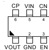
SOT-23-6/TSOT-23-6
