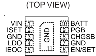
WDFN-10L 3x2
