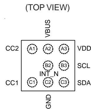
WL-CSP-8B 1.38x1.34 (BSC)
