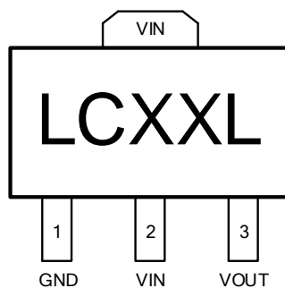
SOT89-3L(L-Type)
